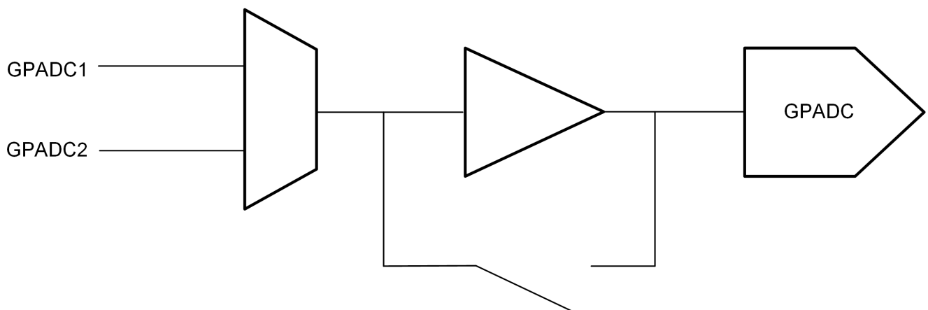
图 8-7. GPADC 路径
