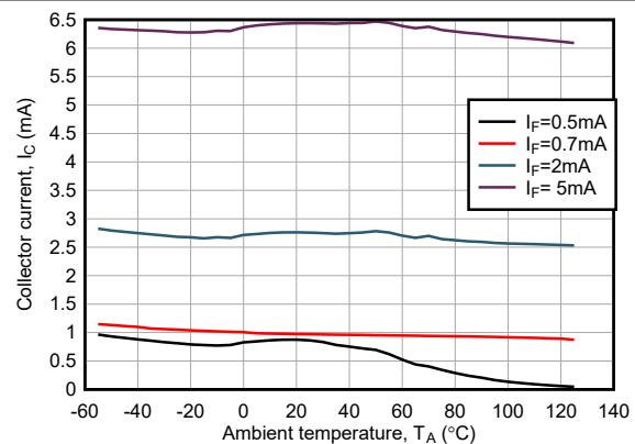
ISOM8110 和 ISOM8115 V_{CE} = 5V
