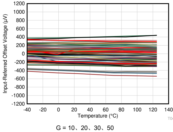
图 7-11. 输入参考失调电压与温度间的关系
