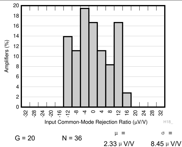
图 7-8. CMRR 的典型分布
