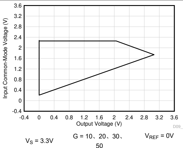
图 7-54. 输入共模电压与输出电压间的关系 (高 CMRR 区域)
