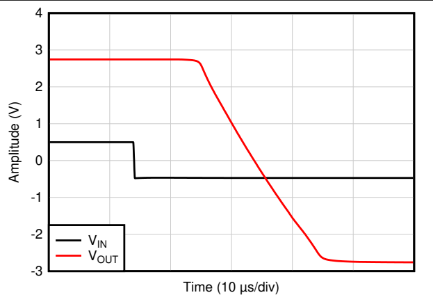
图 7-48. 过载恢复 (下降沿)
