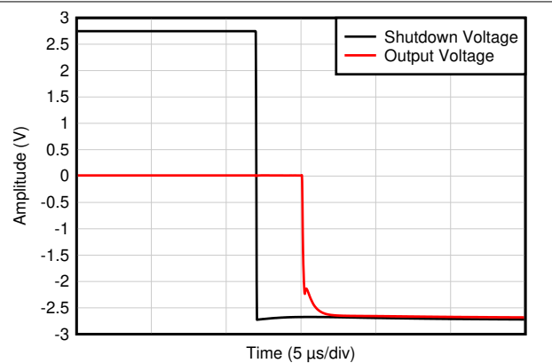
图 7-49. 无相位反转
