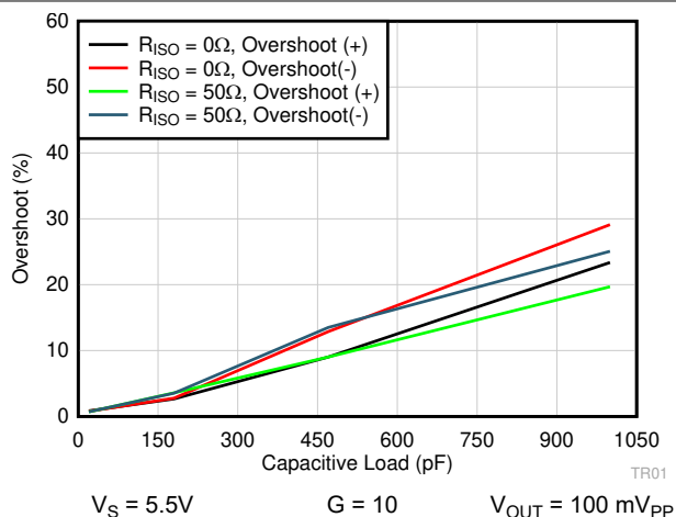
图 7-39. 小信号过冲与容性负载间的关系
