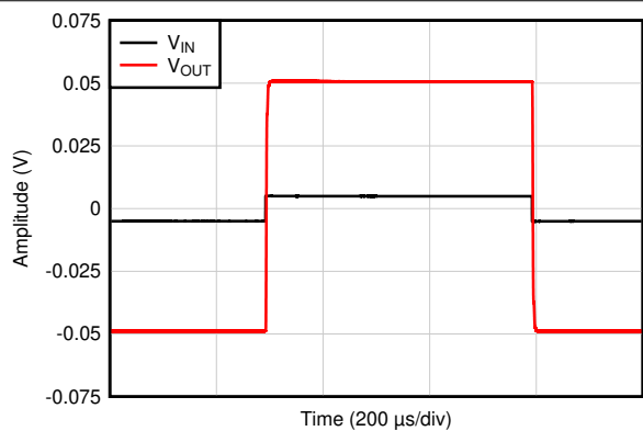
图 7-43. 大信号稳定时间 (上升沿)
