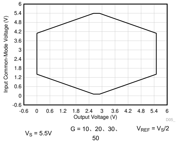
图 8-2. 输入共模电压与输出电压间的关系
