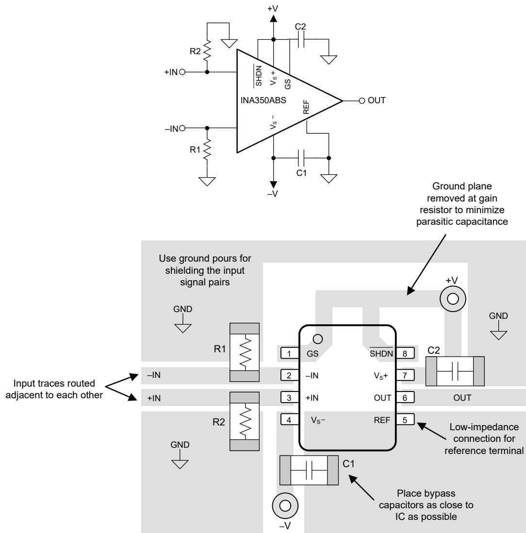
图 9-6. 原理图和相关 PCB 布局示例
