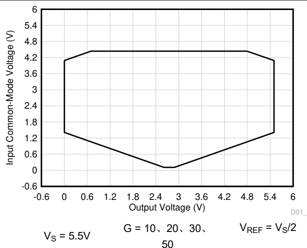
图 7-53. 输入共模电压与输出电压间的关系 (高 CMRR 区域)
