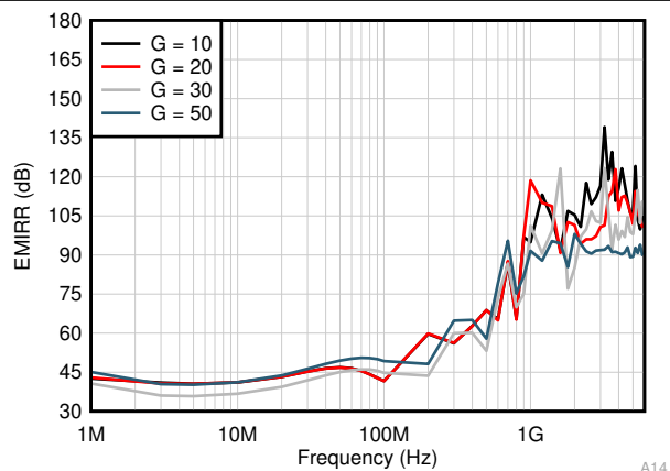
图 7-38. 以同相输入为基准的电磁干扰抑制比 (EMIRR+) 与频率间的关系
