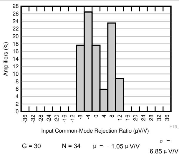
图 7-9. CMRR 的典型分布
