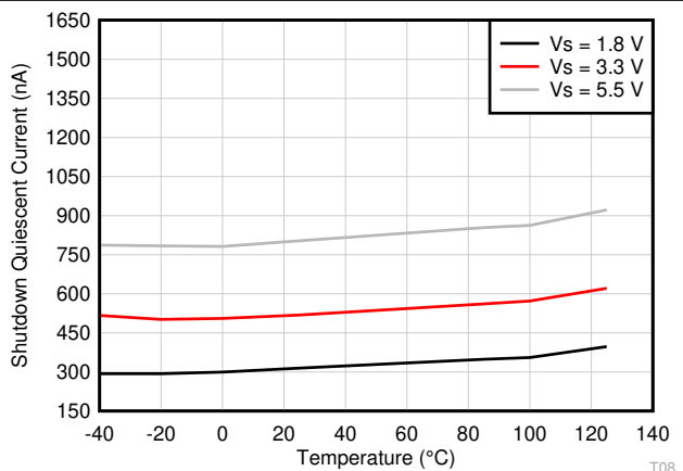
图 7-15. 关断静态电流与温度间的关系
