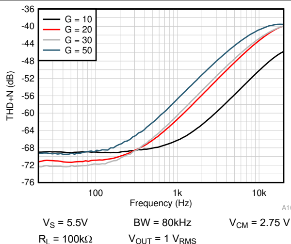
图 7-37. THD + N 与频率间的关系
