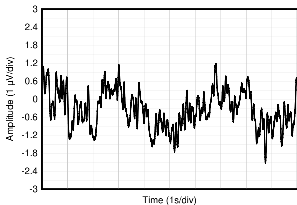
图 7-33. 0.1Hz 至 10Hz 时域电压噪声
