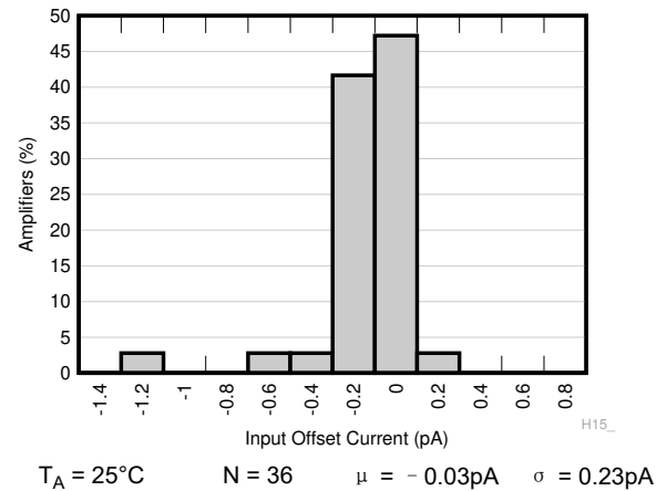
图 7-4. 输入失调电流的典型分布
