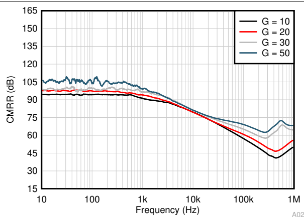
图 7-29. CMRR (以输入为参考) 与频率间的关系
