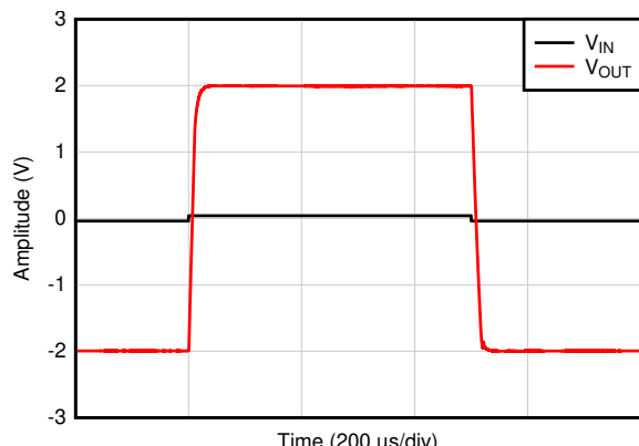
图 7-42. 大信号稳定时间 (下降沿)
