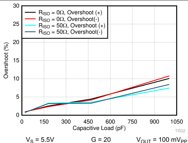
图 7-40. 小信号过冲与容性负载间的关系
