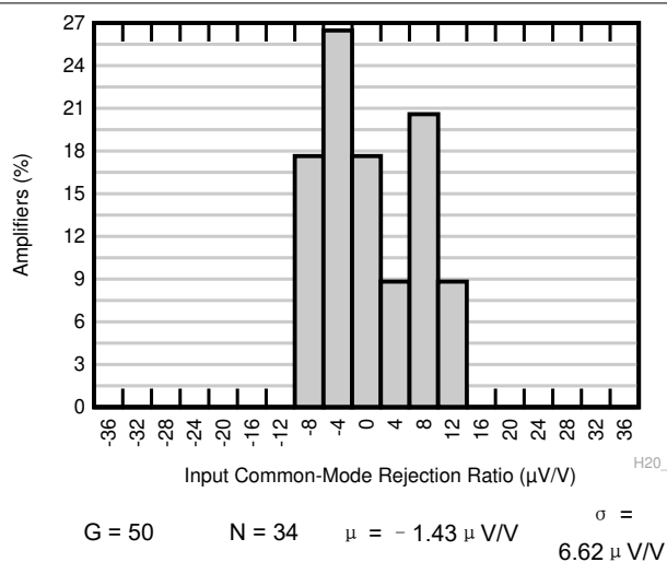
图 7-10. CMRR 的典型分布
