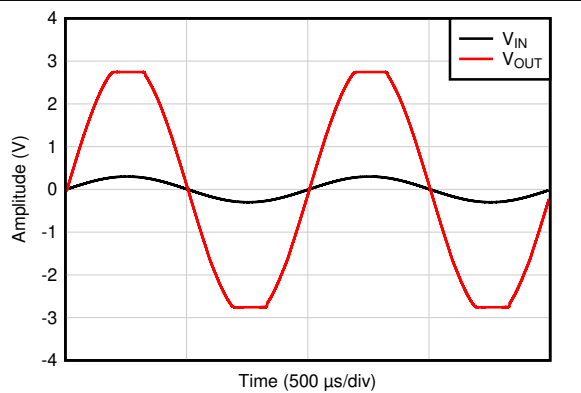
图 7-47. 过载恢复 (上升沿)
