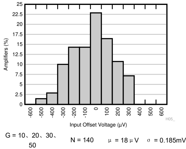
图 7-1. 输入参考失调电压的典型分布
