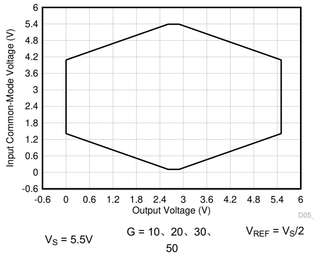
图 7-57. 输入共模电压与输出电压间的关系
