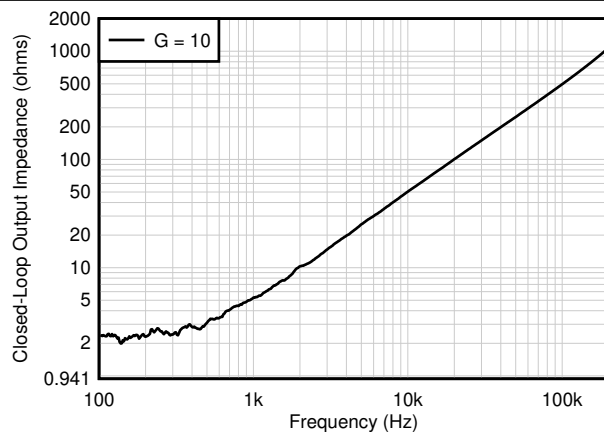
图 7-34. 闭环输出阻抗与频率间的关系
