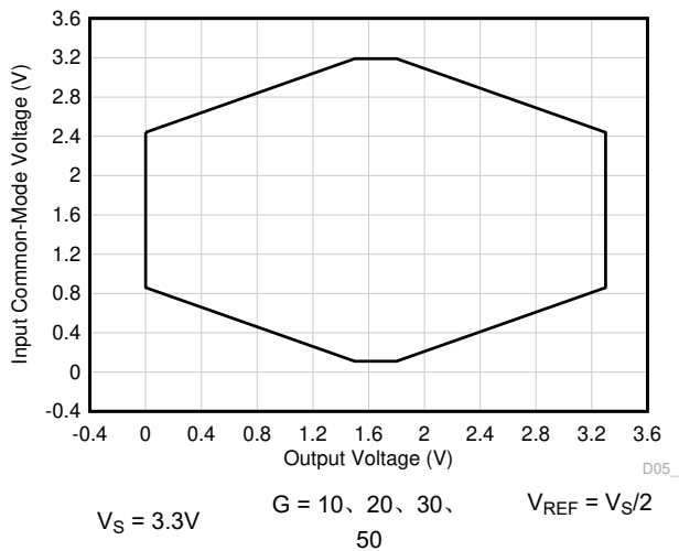
图 7-56. 输入共模电压与输出电压间的关系
