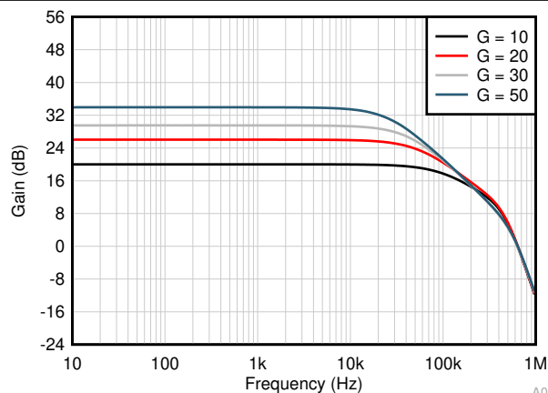
图 7-28. 闭环增益与频率间的关系
