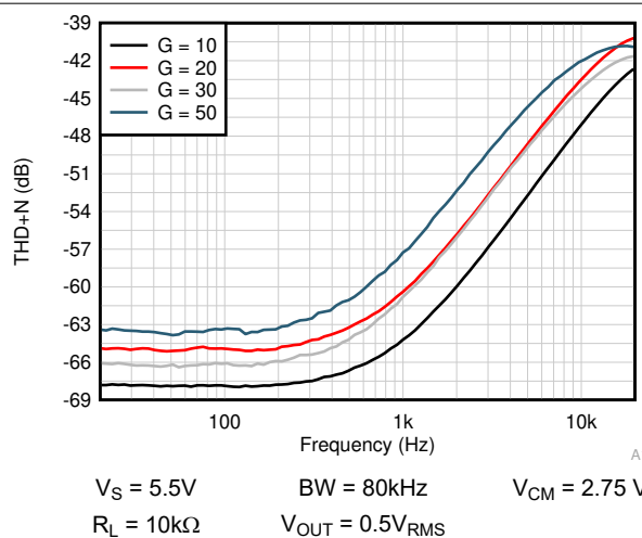
图 7-36. THD + N 与频率间的关系
