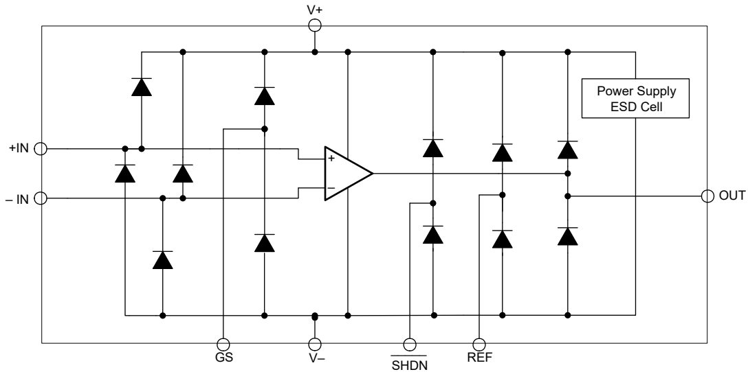
图 8-5. 等效内部 ESD 电路
