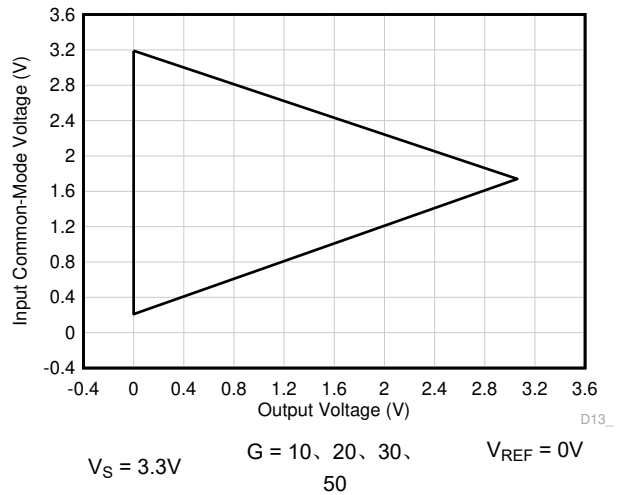
图 7-58. 输入共模电压与输出电压间的关系
