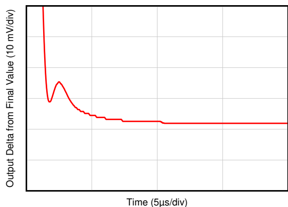
图 7-41. 大信号阶跃响应
