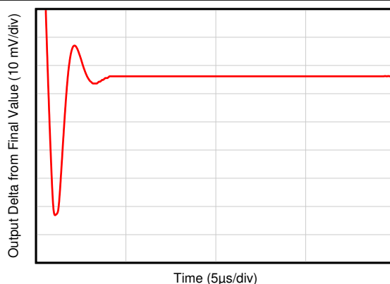
图 7-42. 大信号稳定时间 (下降沿)
