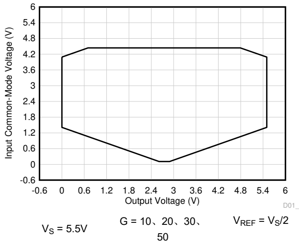
图 8-1. 输入共模电压与输出电压间的关系 (高 CMRR 区域)
