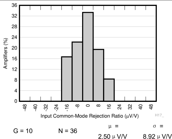
图 7-7. CMRR 的典型分布
