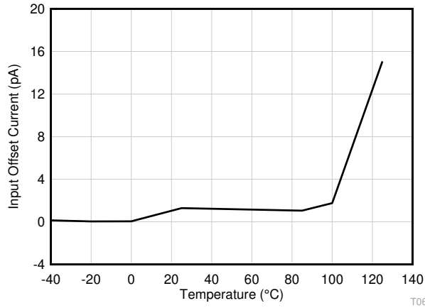
图 7-13. 输入失调电流与温度间的关系
