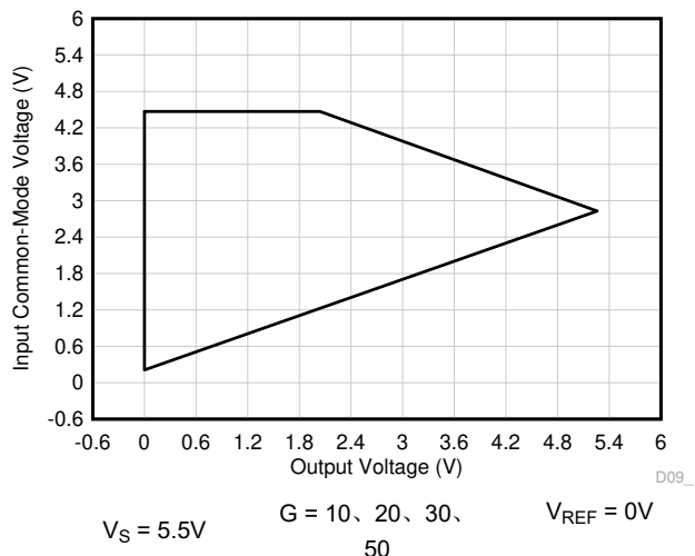
图 7-55. 输入共模电压与输出电压间的关系 (高 CMRR 区域)
