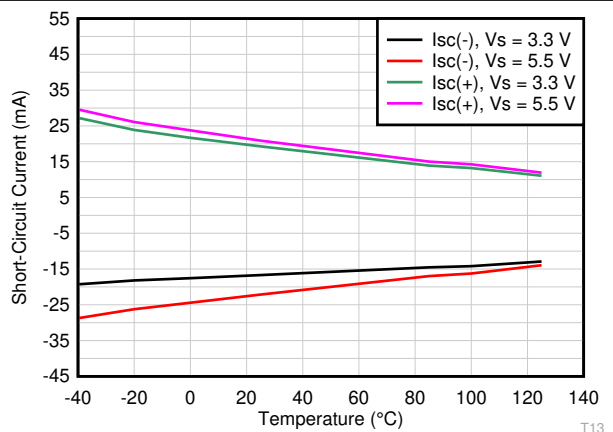
图 7-16. 短路电流与温度间的关系
