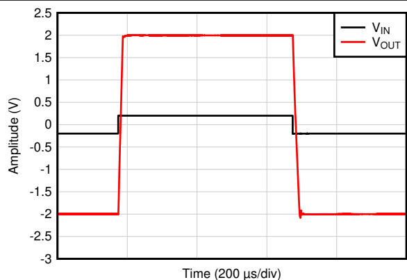
图 7-41. 大信号阶跃响应
