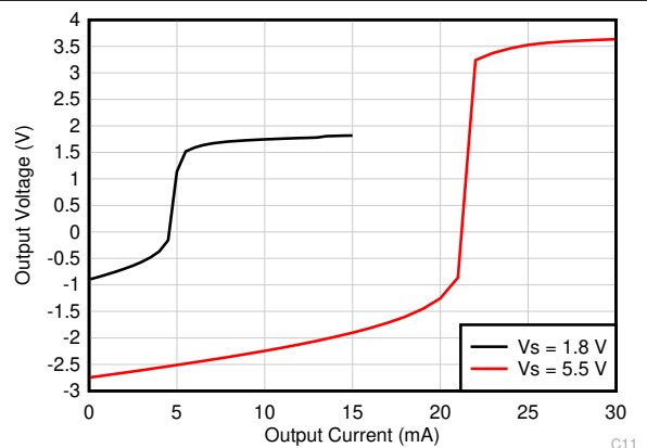
图 7-27. 输出电压与输出电流 (灌电流) 间的关系
