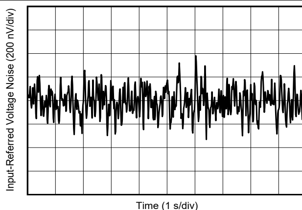
图 6-28. 0.1Hz 至 10Hz 电压噪声
