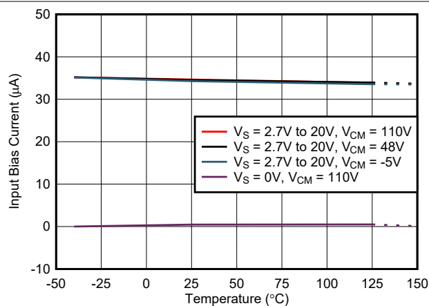
图 6-17. 输入偏置电流与温度间的关系
