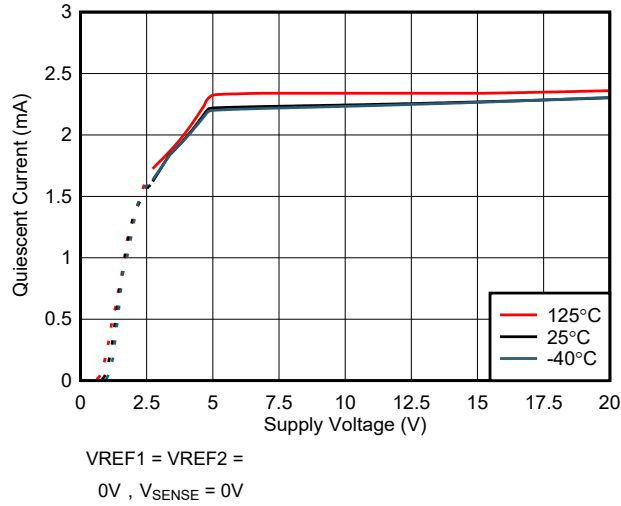
图 6-31. 静态电流与电源电压间的关系
