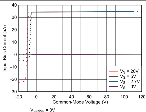
图 6-16. 输入偏置电流与共模电压间的关系
