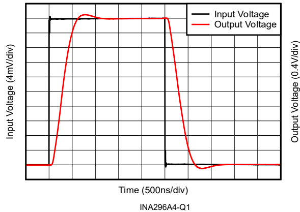
图 6-35. 大阶跃响应
