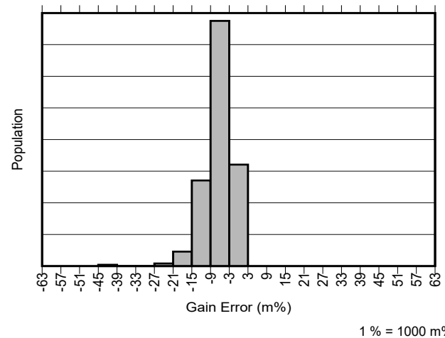
图 6-12. 所有增益 INA296B-Q1 增益误差产生分布图
