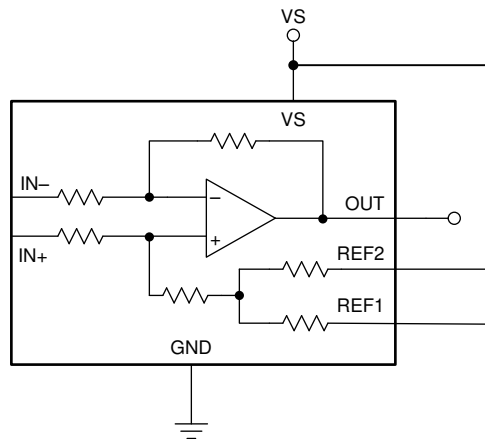
图 7-3. 以 VS 为基准的输出
