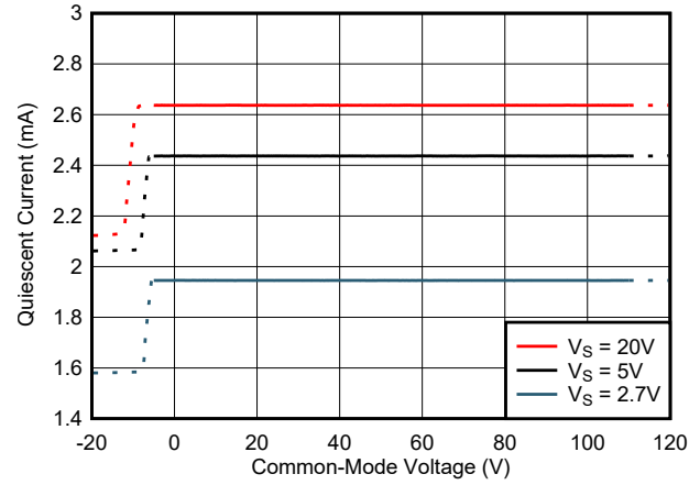
图 6-32. 静态电流与共模电压间的关系
