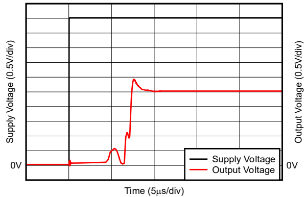
图 6-34. 小阶跃响应
