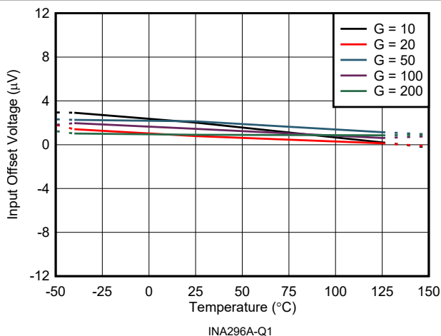
图 6-6. 输入失调电压与温度间的关系
