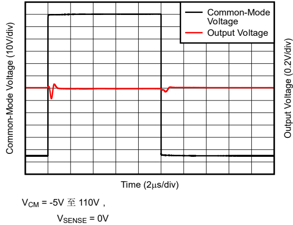
图 6-33. 共模电压快速瞬态脉冲
