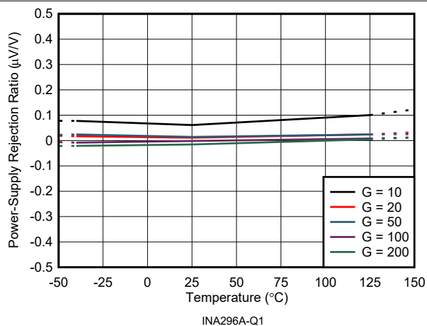
图 6-14. 电源抑制比与温度间的关系
