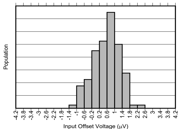
图 6-4. INA296A5-Q1 输入失调电压产生分布图
