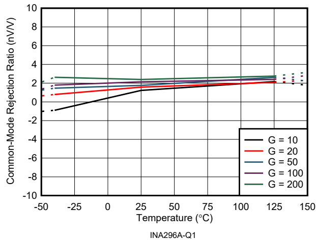
图 6-7. 共模抑制比与温度间的关系
