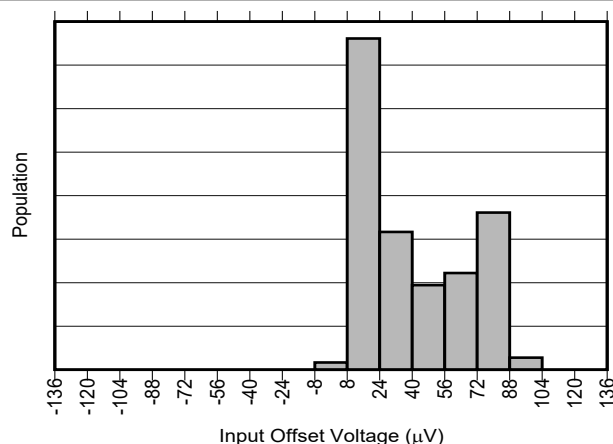
图 6-3. INA296A3-Q1 和 INA296A4-Q1 输入失调电压产生分布图
