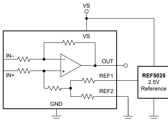
图 7-6. 1/2 外部基准输出
