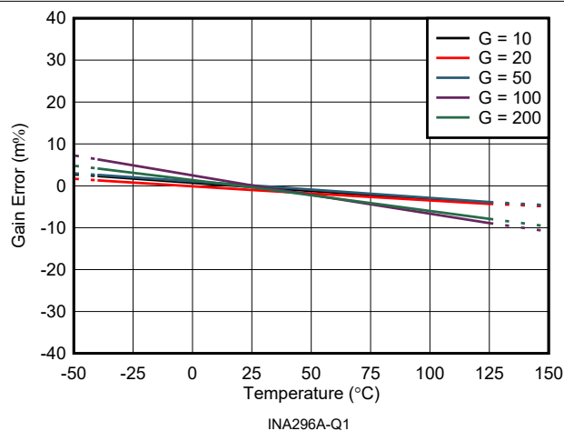
图 6-13. 增益误差与温度间的关系
