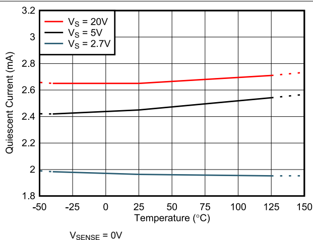
图 6-30. 静态电流与温度间的关系
