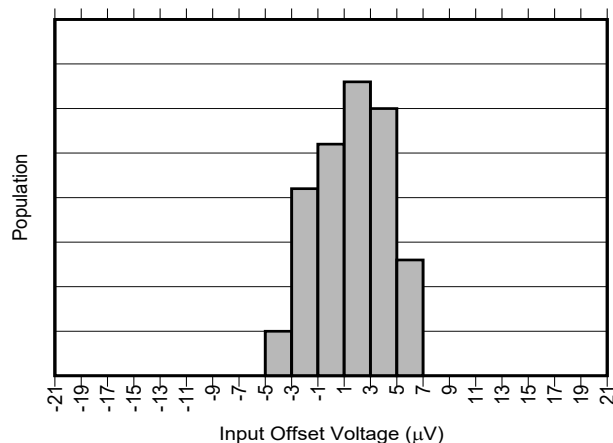
图 6-1. INA296A1-Q1 输入失调电压产生分布图
