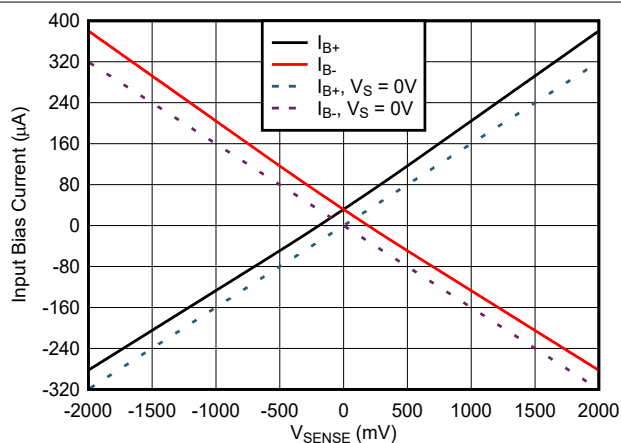
图 6-18. INA241x1-Q1 输入偏置电流与 V_{\text{SENSE}} 间的关系
