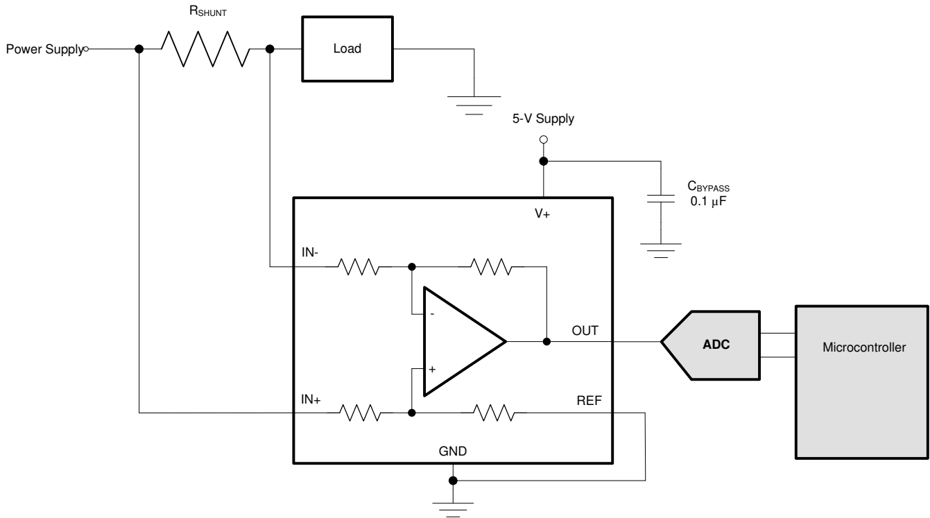
图 6-1. 典型应用
