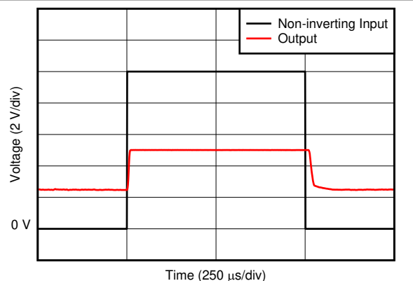
图 6-14. 共模电压瞬态响应
