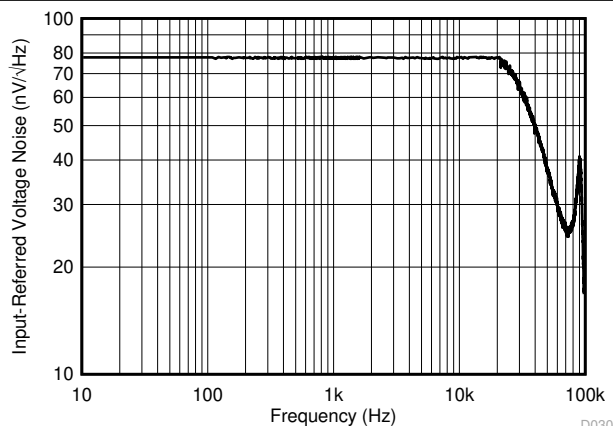
图 6-11. 输入参考电压噪声与频率间的关系
