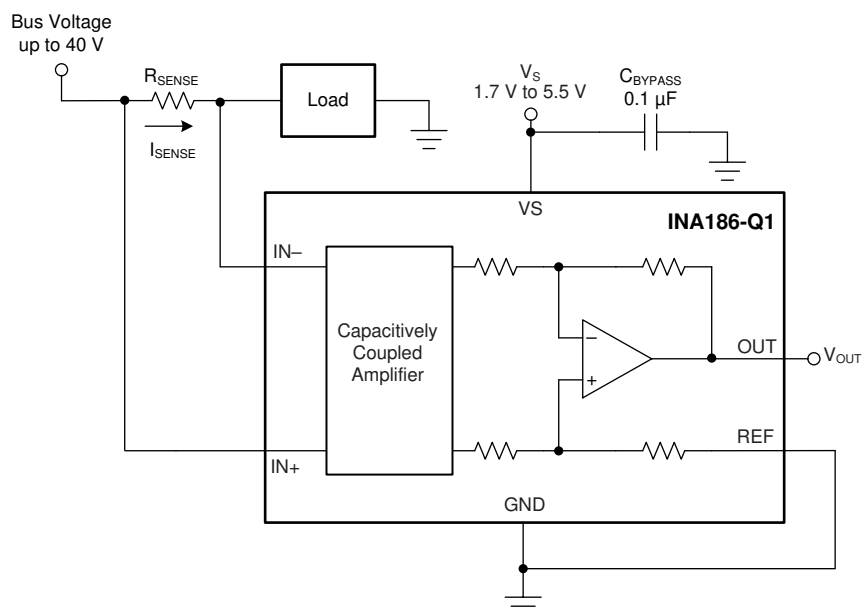
图 7-2. 典型的单向应用
