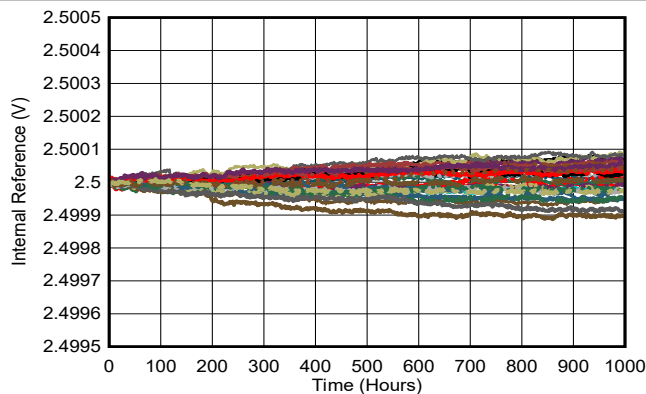
图 5-47. 内部基准电压与时间间的关系 (WQFN)
