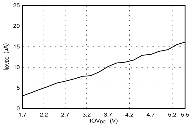
图 5-29. 电源电流 ( I_{IOVDD} ) 与电源电压间的关系
