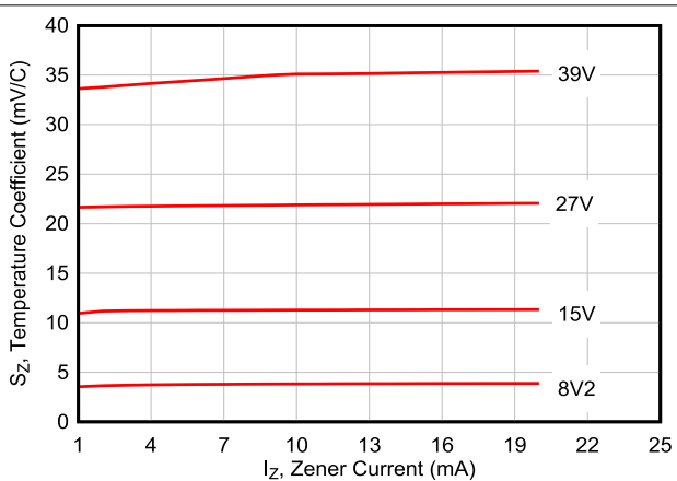
图 5-2. 温度系数
