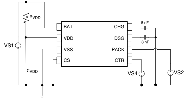
图 8-4. Test Circuit 4
