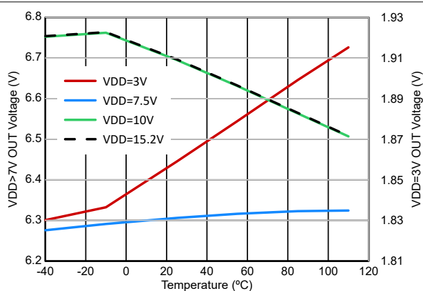
图 6-10. V_{OUT} 与温度间的关系，100 \mu A 负载电流开启 OUT
