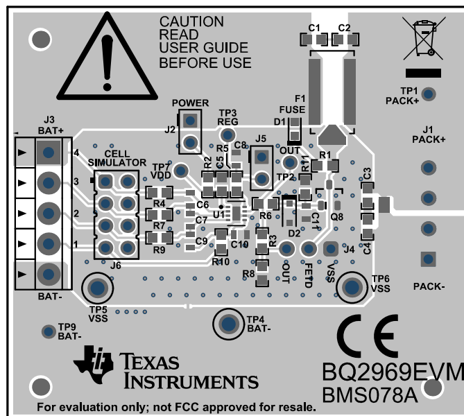
图 10-1. BQ2969 两层电路板布局布线 - 顶层
