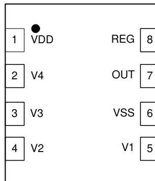
图 5-1. 2-4 节串联电池组 BQ2969 (顶视图)
