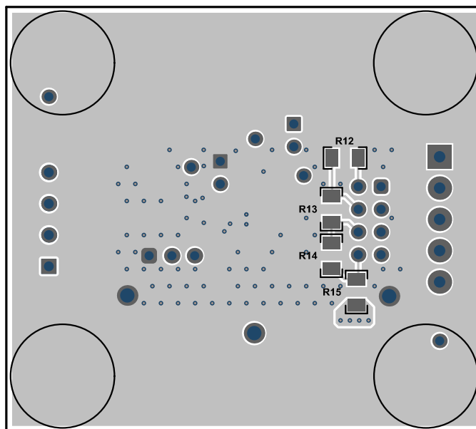
图 10-2. BQ2969 两层电路板布局布线 - 底层
