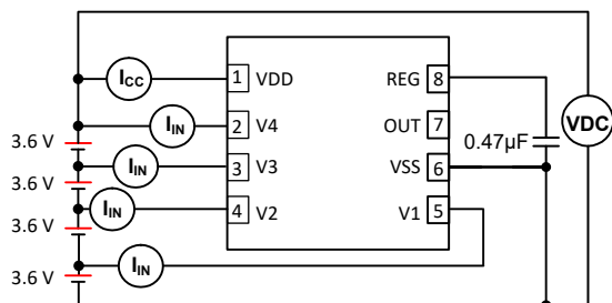
图 7-5. 集成电路电流消耗测试配置
