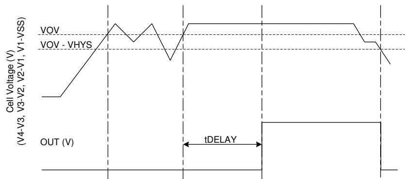
图 7-2. OUT 过压检测时序
