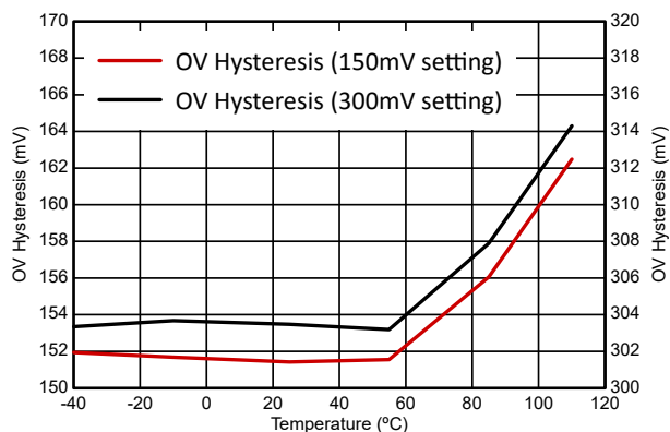
图 6-2. 过压迟滞与温度间的关系
