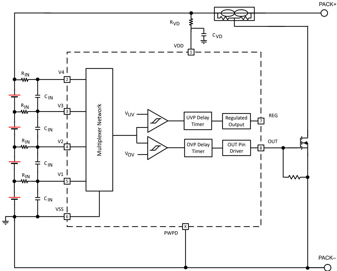
图 7-1. BQ2969 方框图
