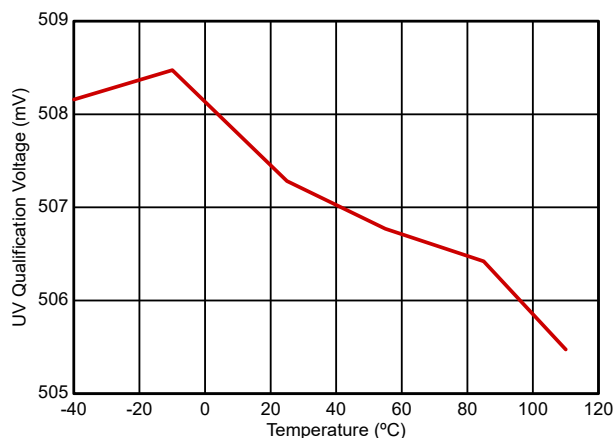
图 6-4. 欠压鉴定电压与温度间的关系
