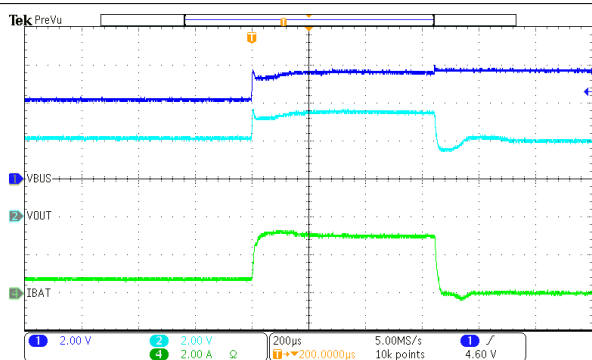
图 9-14. 旁路模式下的 IBATOCP
