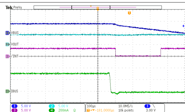
图 9-6. 在旁路模式下拔出适配器
