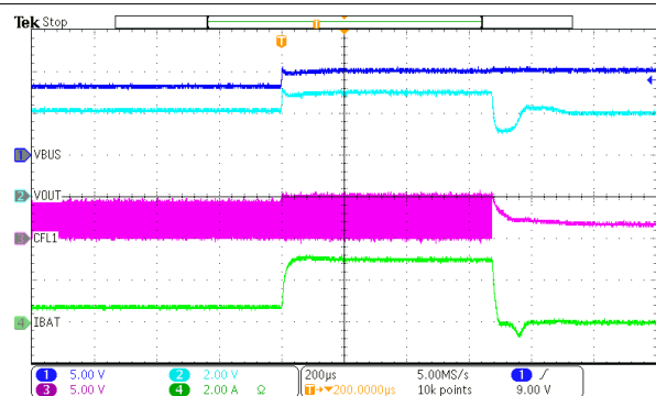
图 9-13. 开关电容模式下的 IBATOCP
