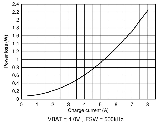
图 7-2. 电池充电功耗与充电电流间的关系，每相 1 x 22 \mu F CFLY 开关频率
