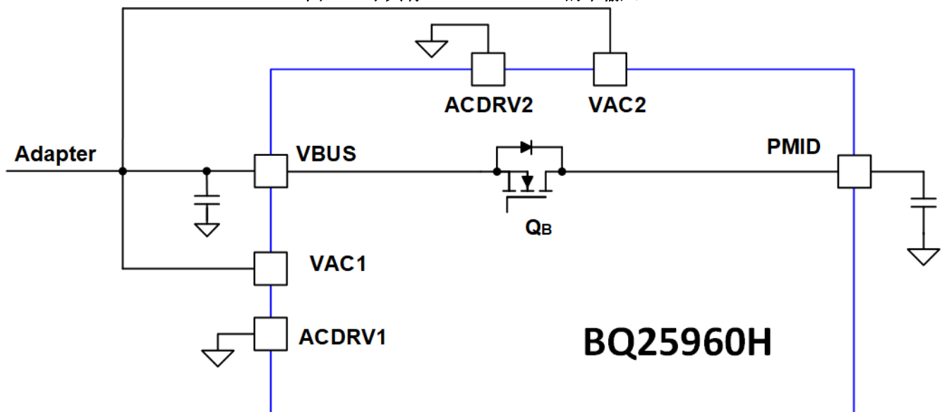
图 8-3. 不具有 ACFET-RBFET 的单输入
