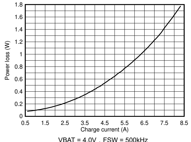
图 7-4. 电池充电功耗与充电电流间的关系，每相 2 x 22 \mu F CFLY
