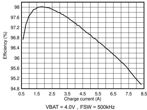
图 7-3. 电池充电效率与充电电流间的关系，每相 2 x 22 \mu F CFLY
