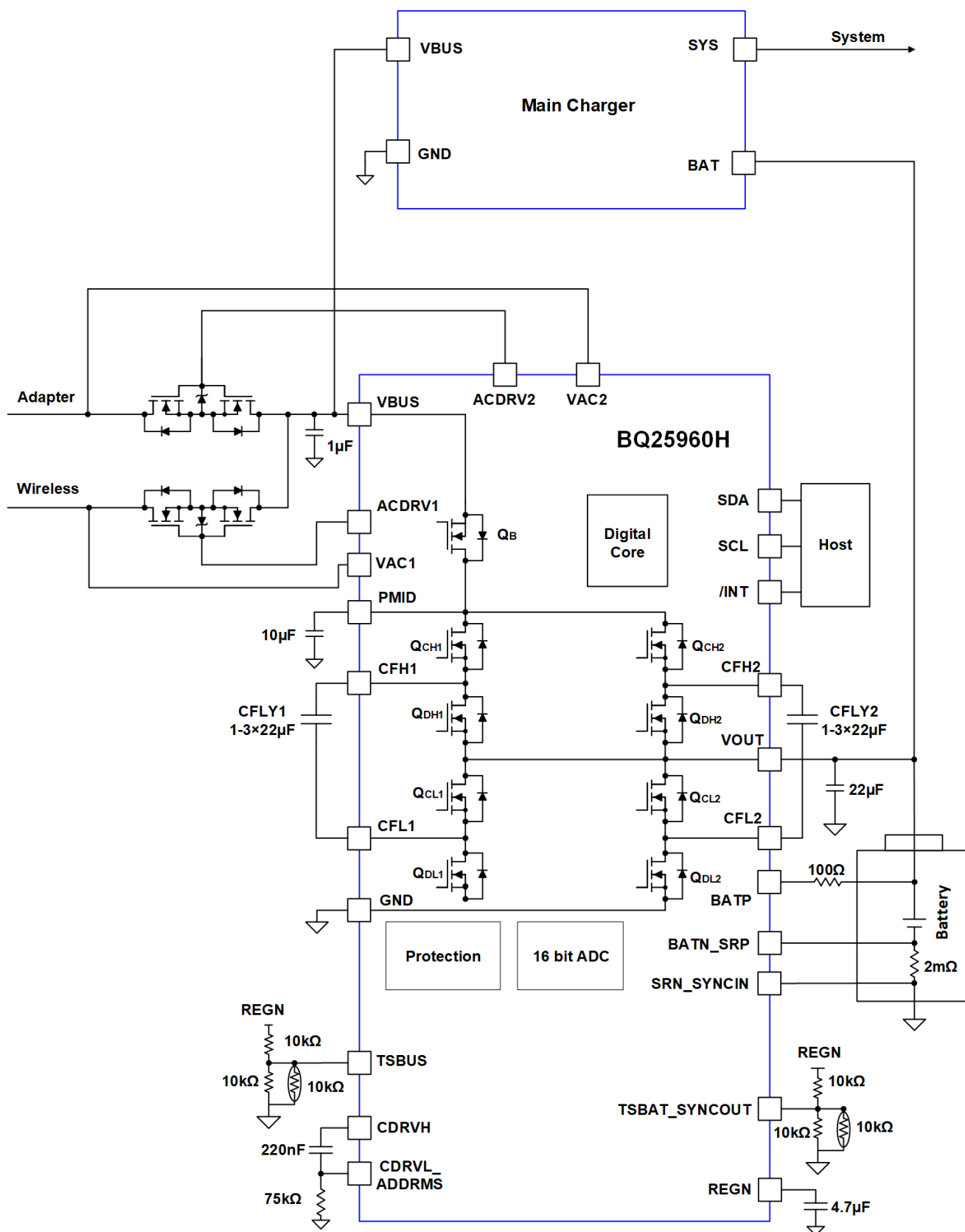
图 9-1. BQ25960H 双输入典型应用图
