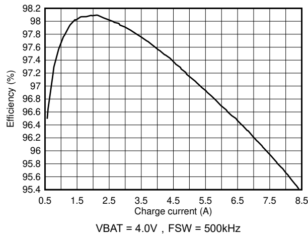
图 7-5. 电池充电效率与充电电流间的关系，每相 3 x 22 \mu F CFLY
