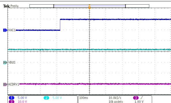
图 9-16. 使用单个 ACFET1 从 VAC1 供电
