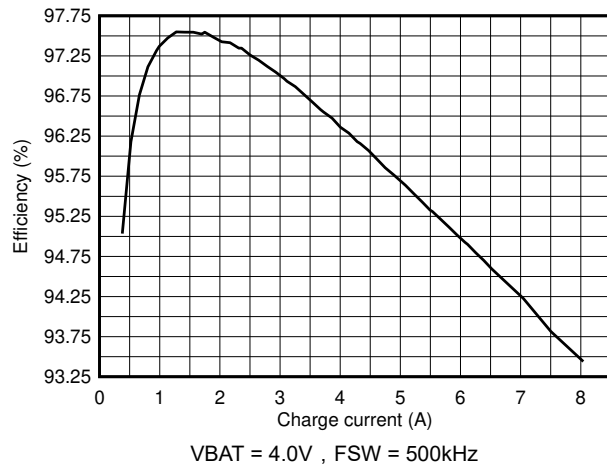
图 7-1. 电池充电效率与充电电流间的关系，每相 1 x 22 \mu F CFLY 开关频率
