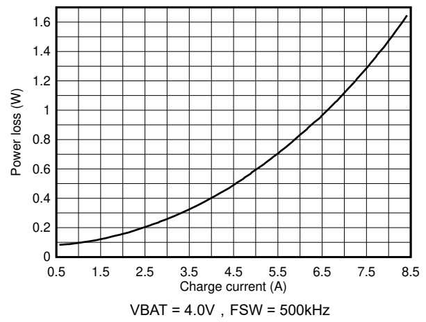
图 7-6. 电池充电功耗与充电电流间的关系，每相 3 x 22 \mu F CFLY
