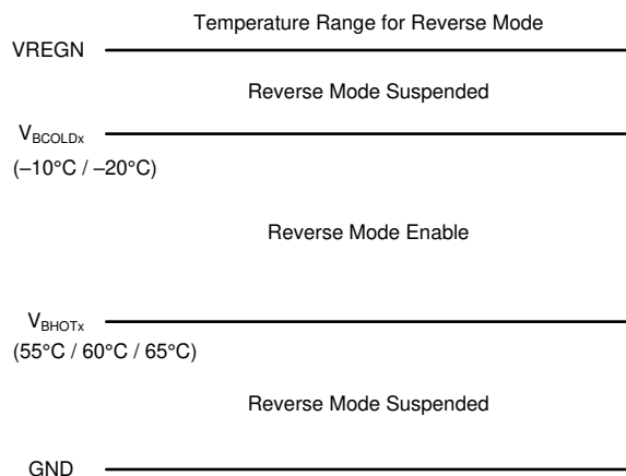
图 7-5. 反向模式下的 TS 引脚热敏电阻检测阈值
