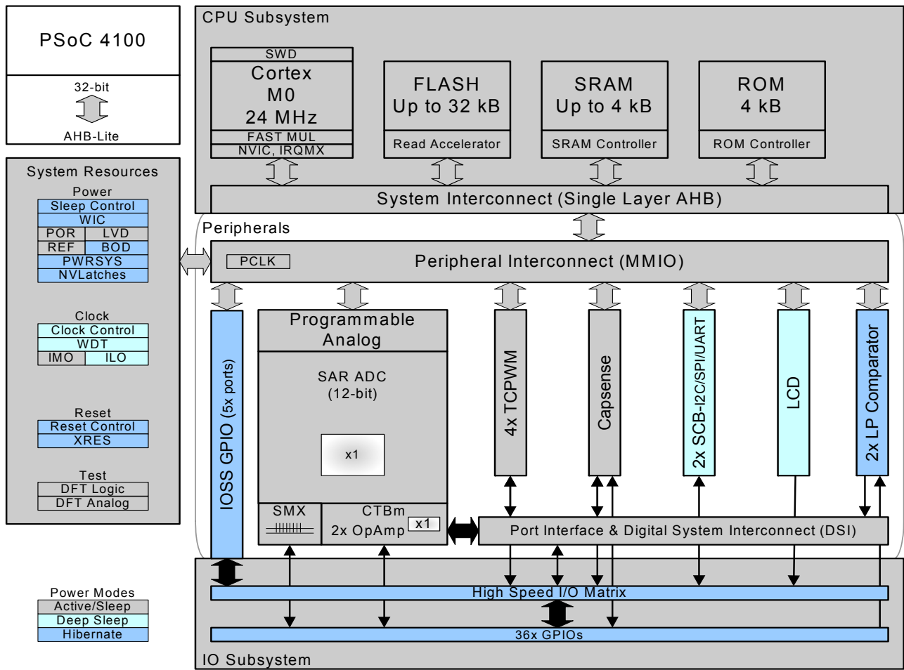
图 2. 框图
